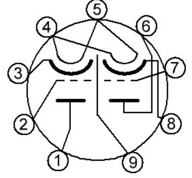
6Н1П/6Н23П/ЕСС88
